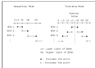
容限模式和顺序模式示意图
