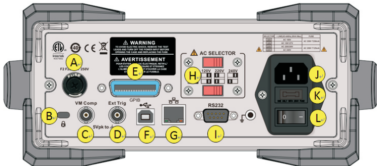
图 1-5 后面板示意图
