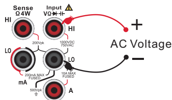
图 2-22 信号周期测量连接示意图
