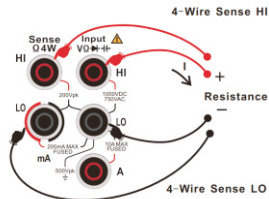
图 2-16 四线电阻测量示意图
