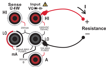
图 2-14 二线电阻测量连接示意图
